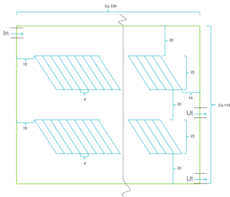
Figur 5 Eksempel på korttidsparkeringsplass med 60 plasser på 16 500 m 2
