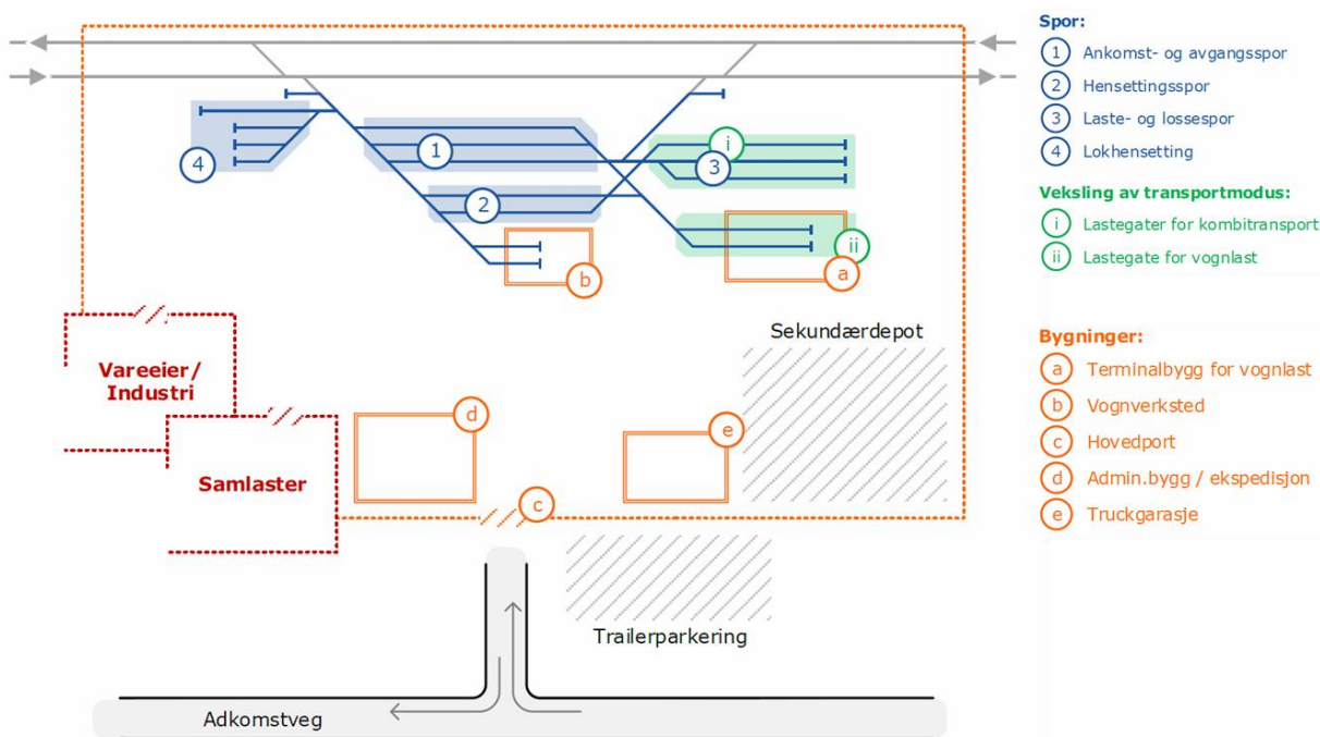
Figur 4 Prinsippskisse intermodal terminal - strategisk rammeverk for terminaler (Jernbaneverket)
