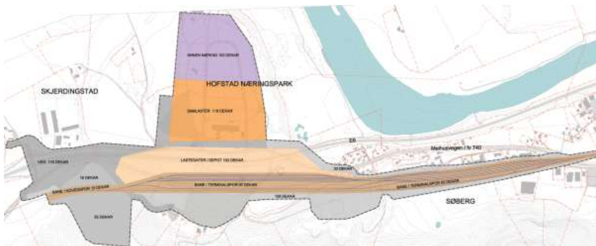
Figur 4-15 Arealplan Sjøberg 2A. Brun areal er bane/spor, lys brun er depot for container, grått er veg, oransje er samlaster og lilla er annen næring.
