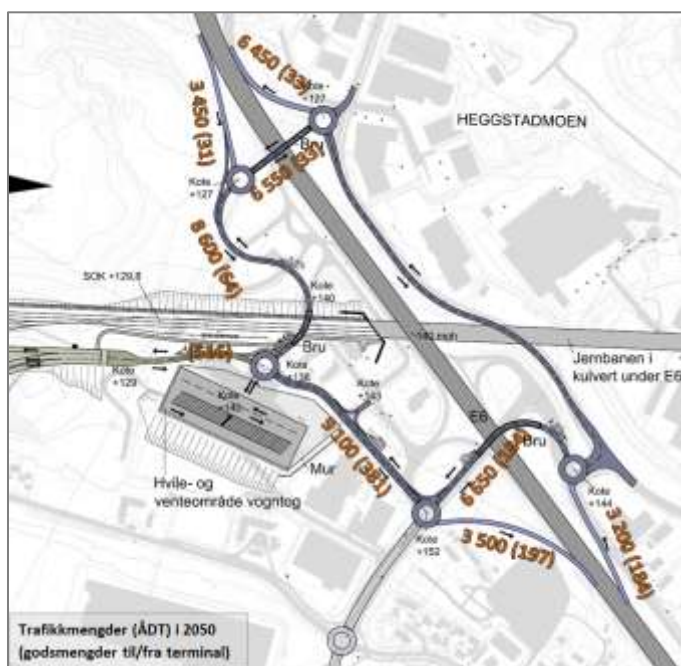
Figur 6-2: Trafikkprognoser for 2050 på rampene til/fra E6 og inn/ut fra terminal på Torgård (samlastertrafikk er ikke inkludert)
