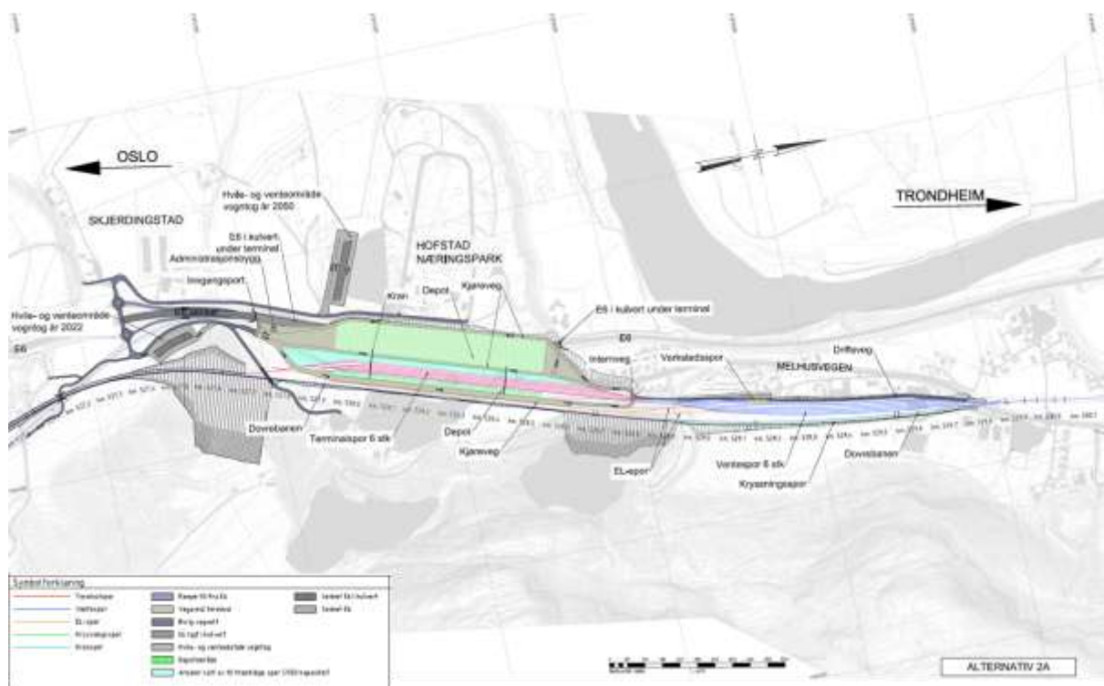
Figur 4-13 Oversiktstegning Alternativ 2a Søberg nord
