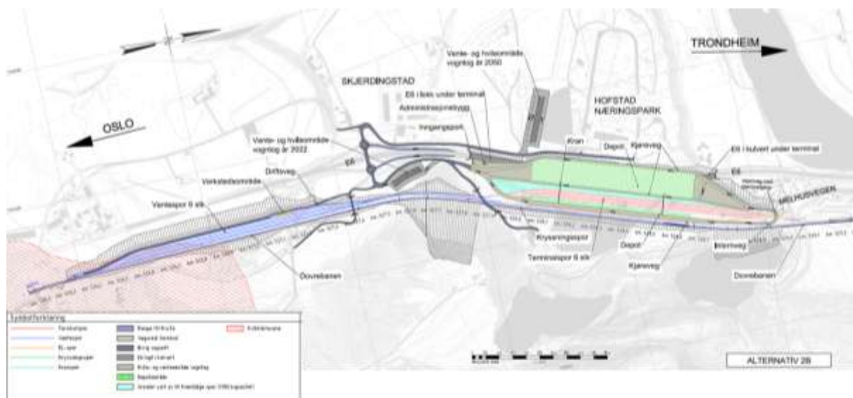
Figur 4-14 Oversiktstegning Alternativ 2b Søberg sør Skjerdingstad
