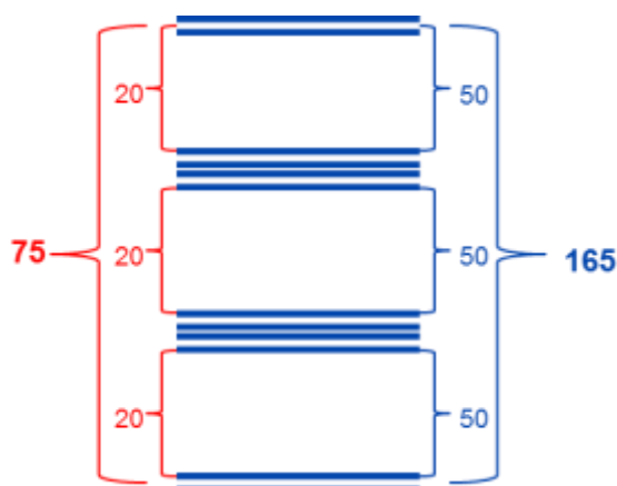
Figur 4-3 Minste og anbefalt bredde for løsningsløsning med reachstackers
