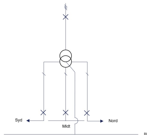
Figur 16: Enlinjeskjema der ladestrekningen er seksjonert i tre deler og hver er tilknyttet ulike faser
