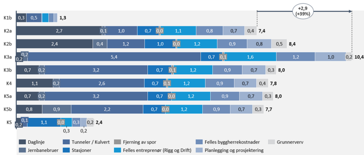
Figur 6 – Nedbrytning av basiskostnaden for alle konsepter eksklusiv omfang knyttet til «Kongsberg – Sandsværmoen» (KS), med vendeanlegg på Kongsberg stasjon hvor dette er aktuelt.
