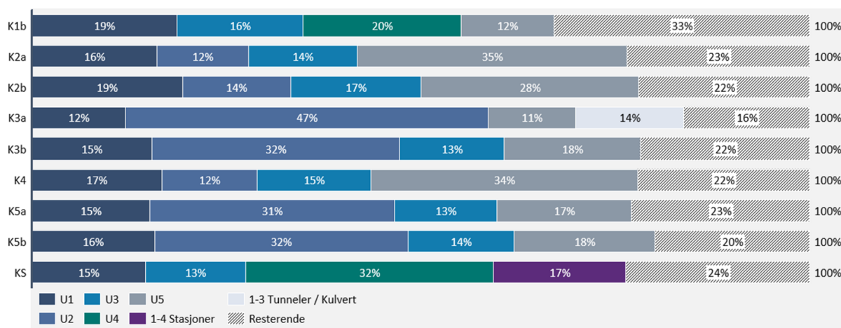
Figur 10 – Kostnadsposter og usikkerhetsdrivere som bidrar mest til den totale usikkerheten i konseptene eksklusiv opsjon Kongsberg – Sandsværmøen, med vendeanlegg på Kongsberg stasjon for konsepter hvor dette er relevant.
