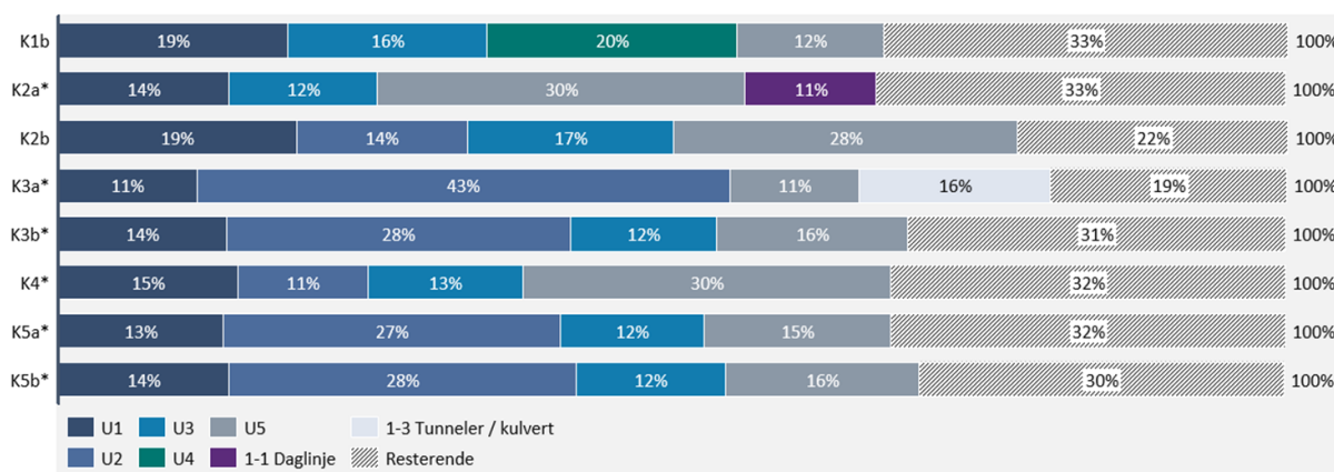
Figur 11 – Kostnadsposter og usikkerhetsdrivere som bidrar mest til den totale usikkerheten i konseptene inklusiv opsjon Kongsberg – Sandsværmøen for konsepter markert med *
