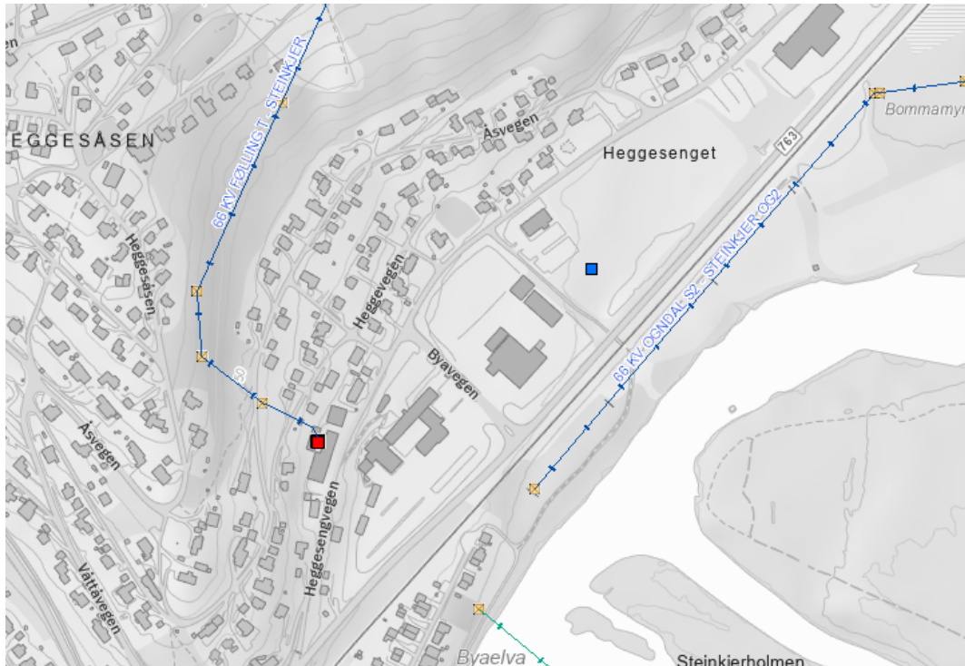
Figur 2. 66 kV Steinkjer transformatorstasjon (rød firkant) og konsesjonssøkt omformerstasjon (blå firkant)
