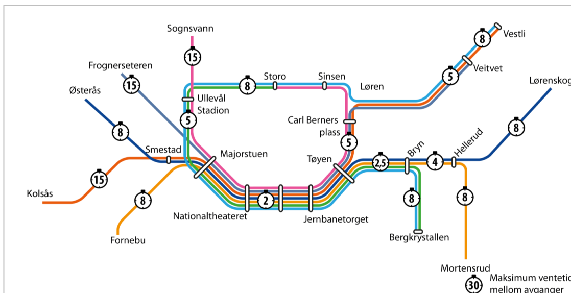
Figur 6-3 Overordnet tilbudskonsept for metro i Nullalternativ+. Makstid mellom avganger i minutter. Illustrasjonen viser det tilbudskonseptet som er beregnet i transportmodellen.
