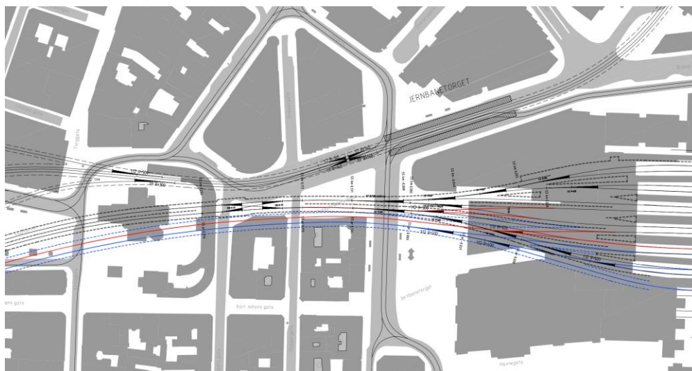
Figur 89: Oversiktstegning Oslo S-Kirkeristen med ensidig utvidelse av Trakta
