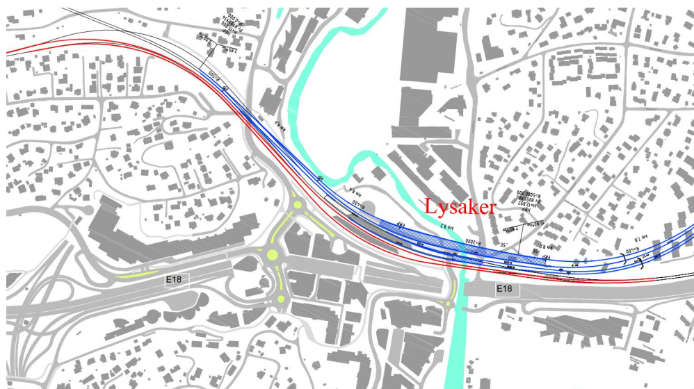
Figur 102: Utvidelse av Lysaker stasjon. Blå farge er regiontog og rød farge er lokalto
