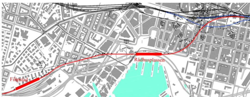
Figur 65: Oversiktstegning S-bane Oslo S-Rådhusplassen-Filipstad
