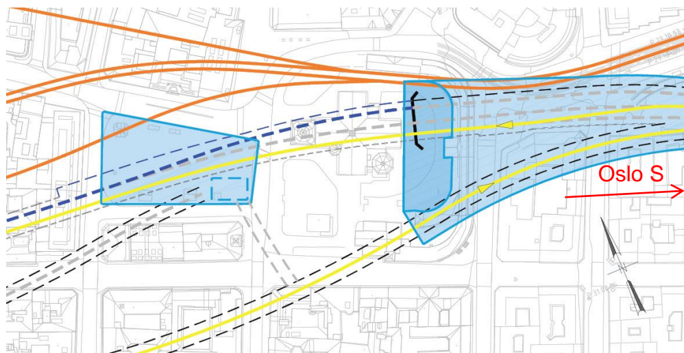
Figur 24: Fase 2, bygging av ny tunnel for utgående tog
