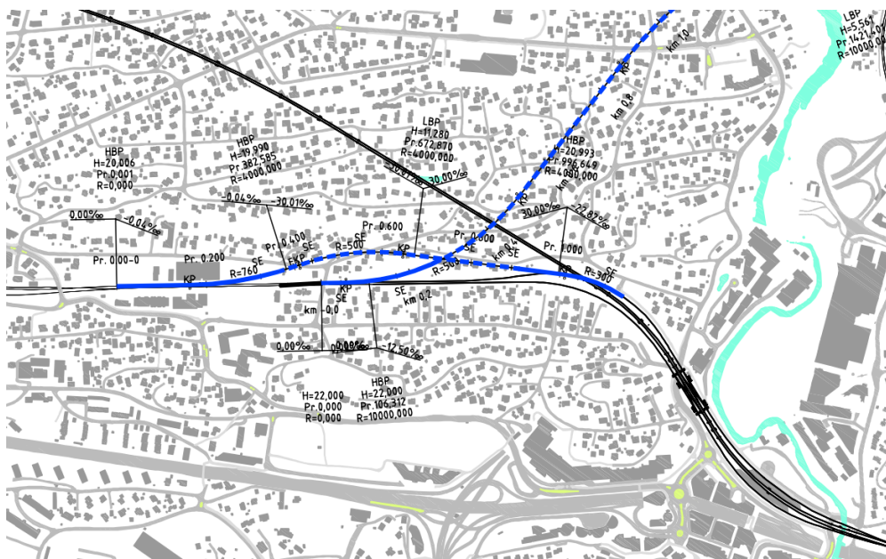
Figur 122: Oversiktstegning godstogtrase Stabekk/Lysaker
