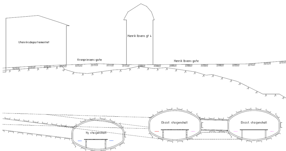
Figur 38: Figuren viser snitt av ny stasjonshall for inngående spor til venstre, og eksisterende stasjonshaller på Nationaltheatret. Eksisterende og ny adkomsttunnel for bygging og rømningstunnel er vist
