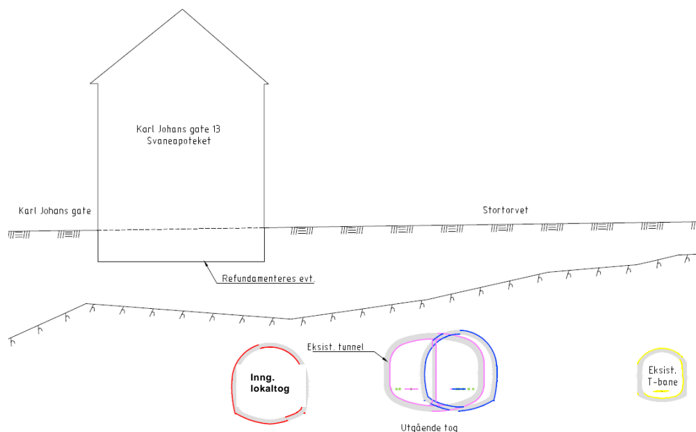
Figur 30: Figuren viser snitt ved Stortorvet av tunnel for inngående lokaltog (rødt), og utgående regiontog (blått) nesten sammenkoblet med eksisterende tunnel. Liten bergoverdekning med behov for forsterkning over berg og evt. refundamentering av bygninger
