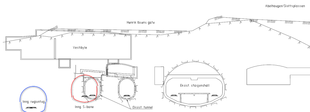
Figur 37: Figuren viser snitt av tunnel for inngående spor ved passering under vestibylen for Nationaltheatret stasjon. Inngående lokaltog (rødt) greiner av fra eksisterende spor. Til høyre stasjonshallen for utgående tog, og helt til høyre P-anlegg i gamle tilfluktsrom under Abelhaugen
