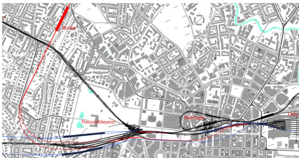
Figur 64: Oversiktstegning S-bane Nationaltheatret-Bislett med jernbanetrasé for regiontog
