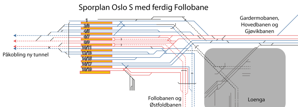
Figur 73: Sporplan Oslo S med påkobling av Follobanen og tilkobling til eventuell ny tunnel.
