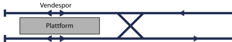
Figur 66: Vending på vendespor ved plattform. En slik løsning har for jernbane kapasitet opp til 3 tog/spor/time. For T-banen kan det vendes opp til 8 T-banetrogner/spor/time. Kilde: [64]
