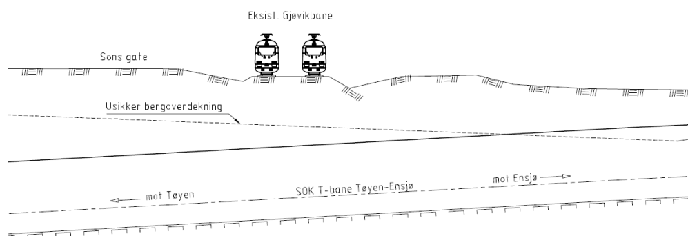
Figur 23: Kryssing under Gjøvikbanen med usikker bergoverdekning.
