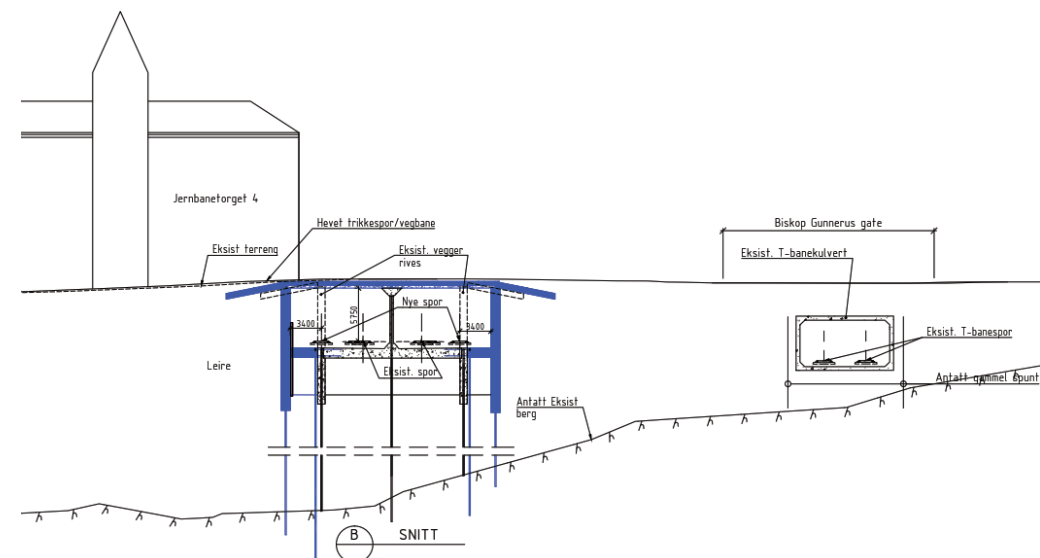
Figur 33: Snitt B under Strandgata
