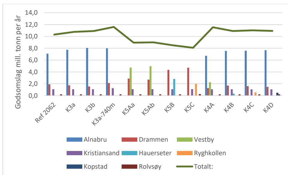
Figur 3.4 Godsomslag jernbaneterminaler Oslofjordområdet 2062 for alternative konsepter (millioner tonn per år).
