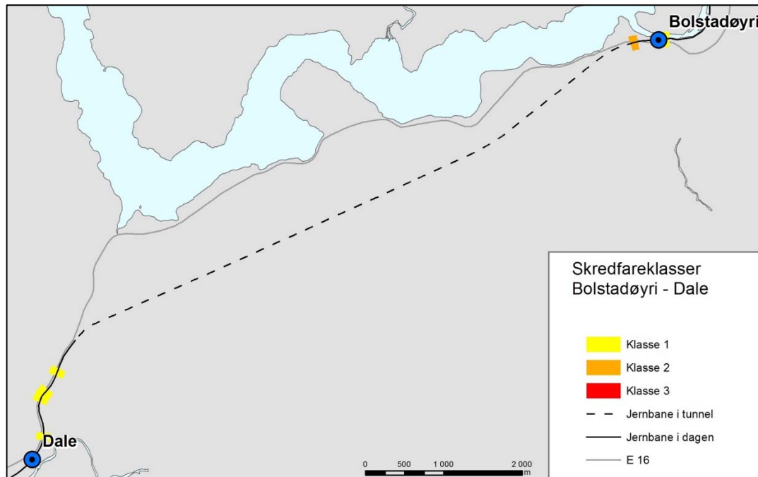
Figur 9: Skredfare Bolstadøyri - Dale
