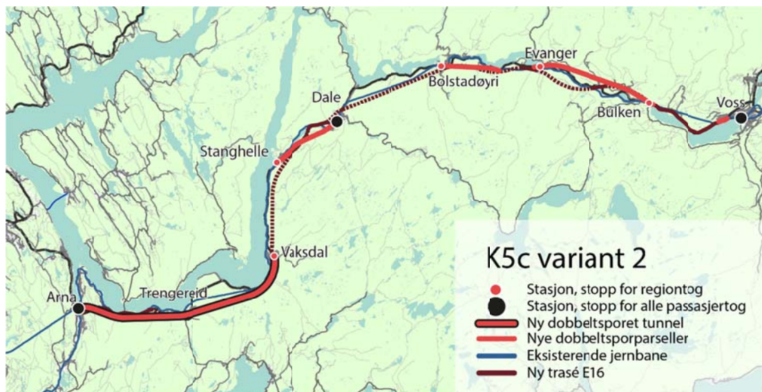
Figur 17: Alternativ K5c variant 2: Dobbeltspor Bergen - Vaksdal, dobbeltsporsparseller
